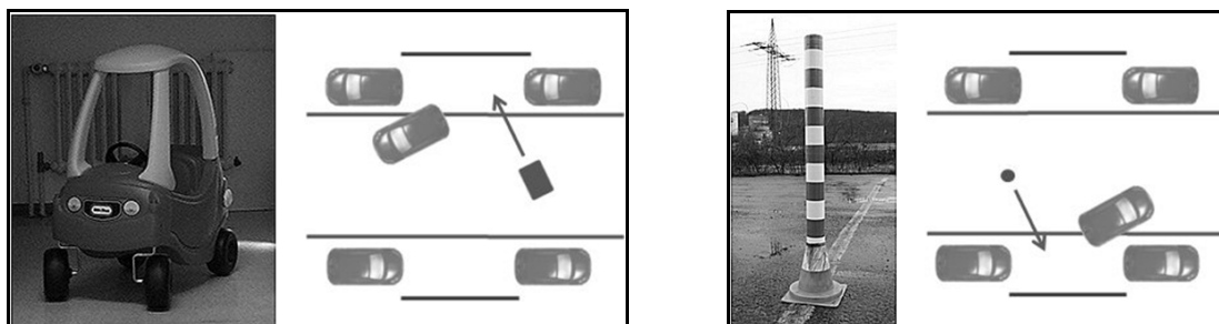
Abbildung 2: Hindernis „Bobbycar“ (links) bzw. „Pfosten“ (rechts) jeweils mit schematischer Darstellung der Situation auf dem Testgelände.
